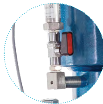
Porta para Transdutor de Pressão Integrado
