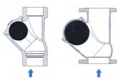
INSTALAÇÃO VERTICAL
